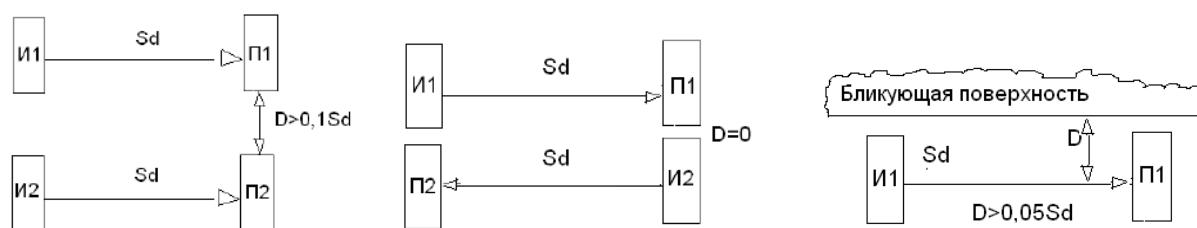
Рис. 5 Варианты установки барьеров
